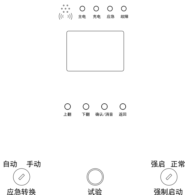
图 6 操作面板图
