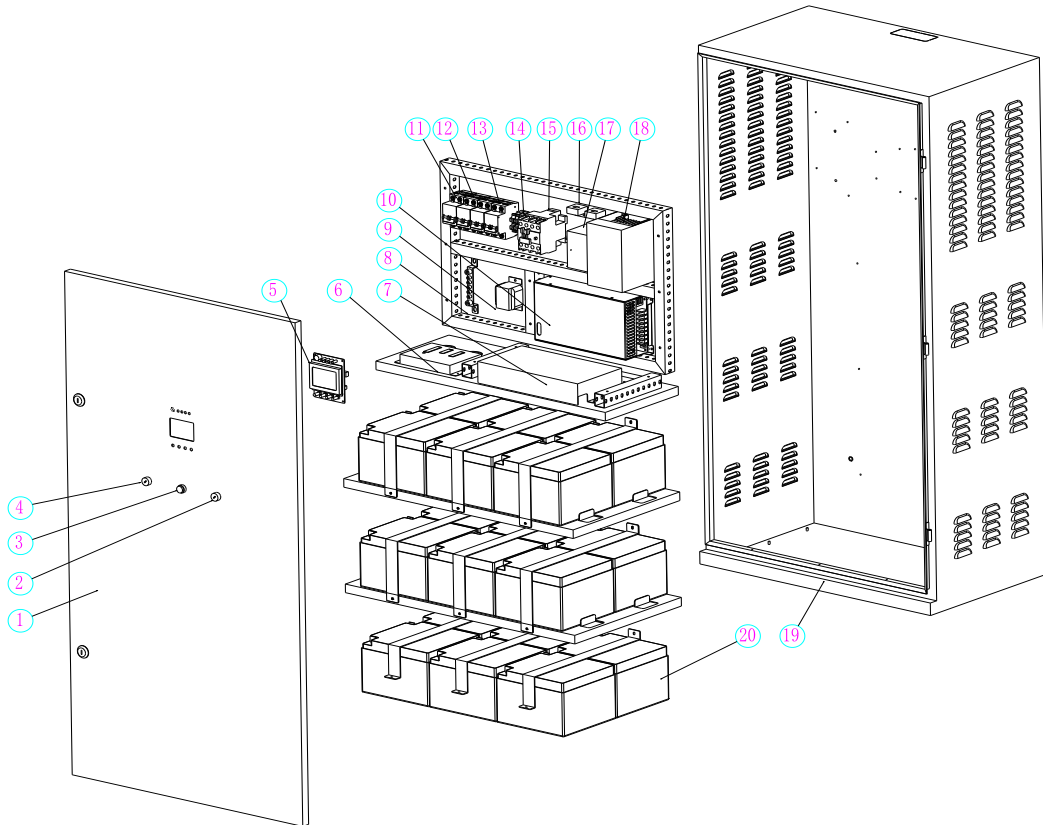
图 2 结构图
