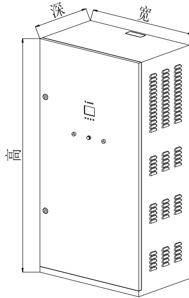
图 1 外形图
