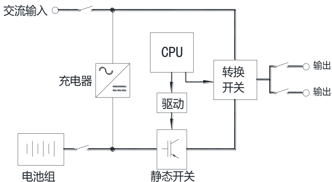
图 3 工作原理图
