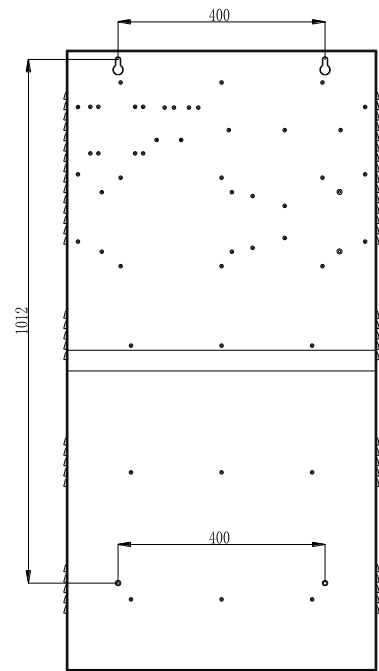
图 4 安装孔距图
