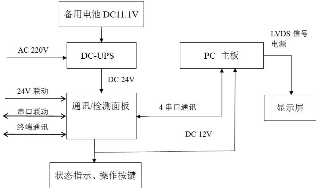
图 3 产品工作原理图
