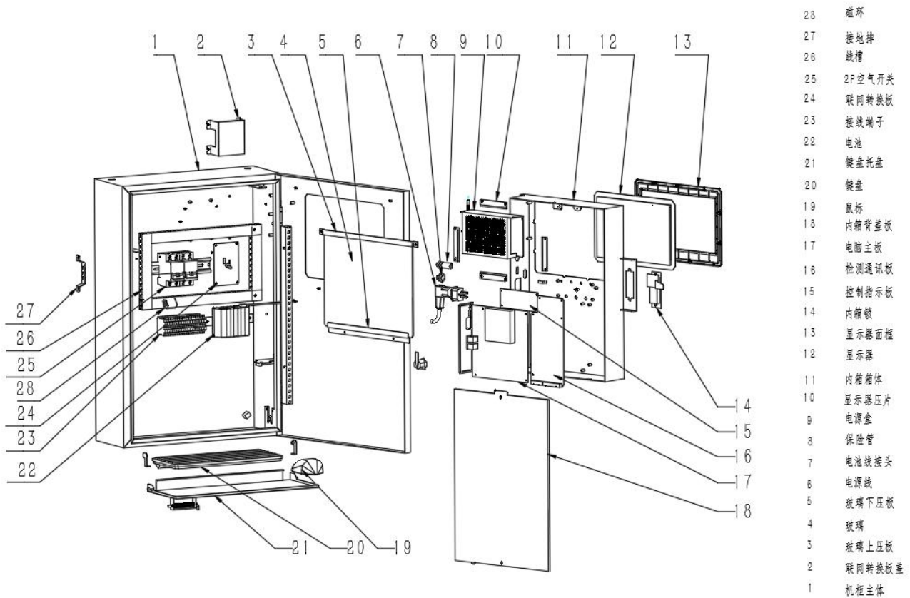
图 1 产品外形图
