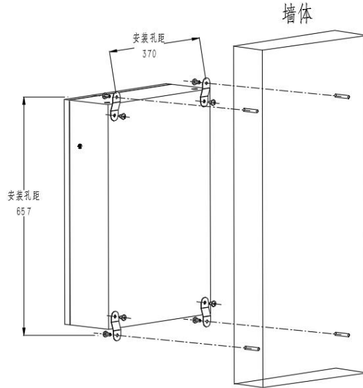
图 4 应急照明控制器安装示意图
