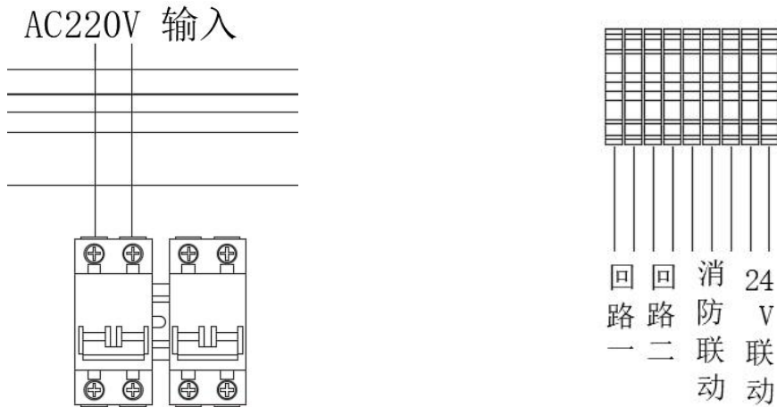
图 5 应急照明控制器接线示意图
